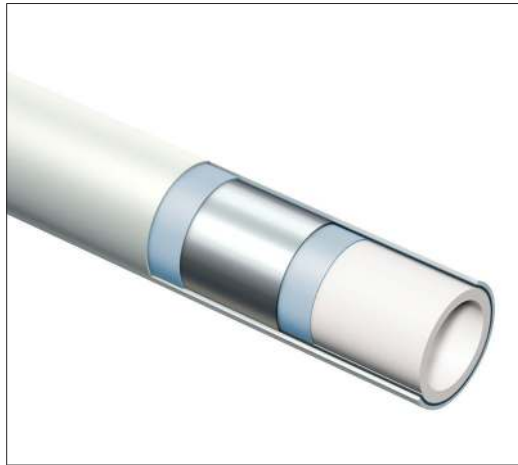
TECEflex Teava multistrat
