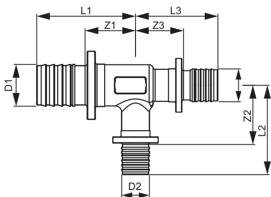
TECEflex teu redus
