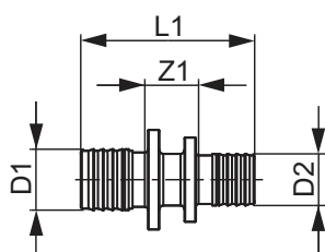
TECEflex niplu redus
