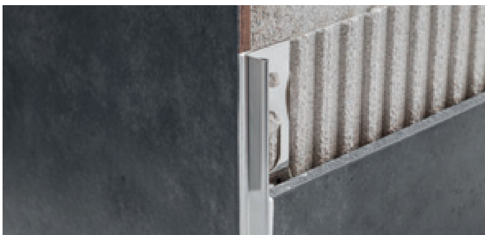
AI/10 stainless steel AISI 304 - DIN 1.4301
