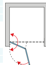
SOLF1 G + V.SOL
