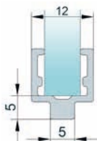
CONCEPT 2x STR4P + VT90 Profil șlefuit lucios (50), Sticlă securizată cu decor crom 62
