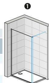
D22WI1 cu bară stabilizatoare
