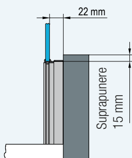
Detaliu A vedere frontală:
